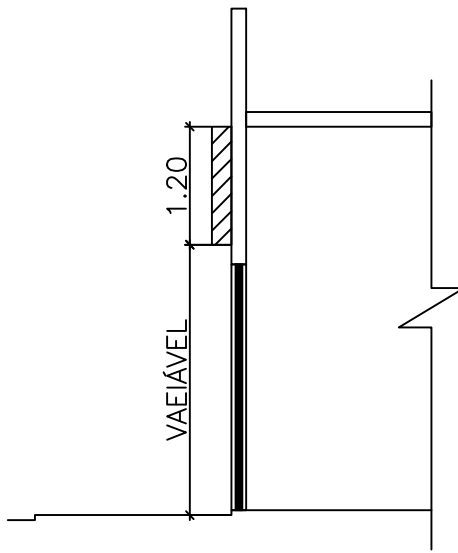
CORTE AA
