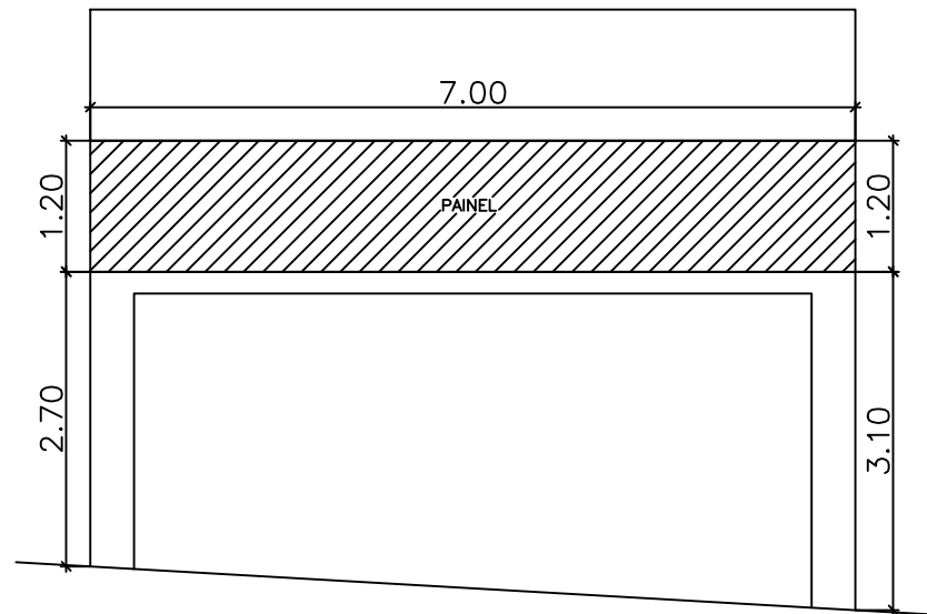
ELEVAÇÃO
