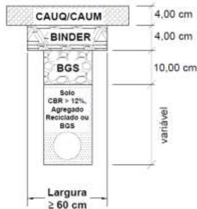
FIGURA 1A VALA - Tráfego Leve Seção Tipo 1
